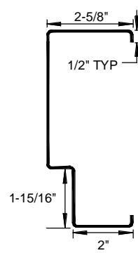
JAMB DETAIL
